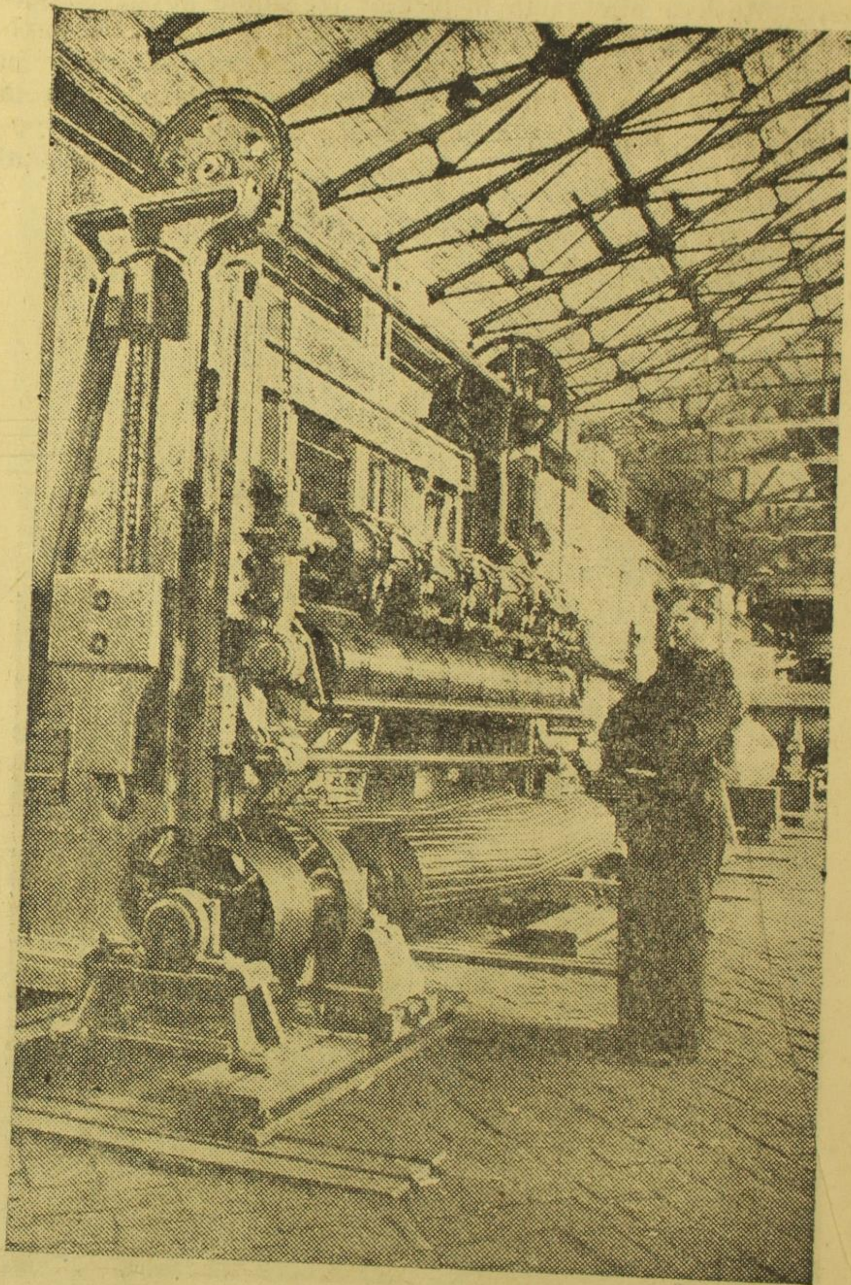
Zavod imena »Druga pjetoljetka« u Lenjingradu izradjuje mašine za rezanje hartije. Na ovoj mašini za rezanje dostiže se brzina od 500 metara izrezane hartije u minuti.
